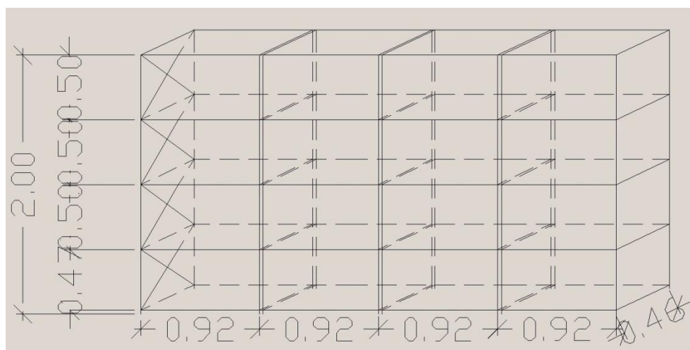
Σχήμα 6. Κατασκευή ΣΤ (dexion)
