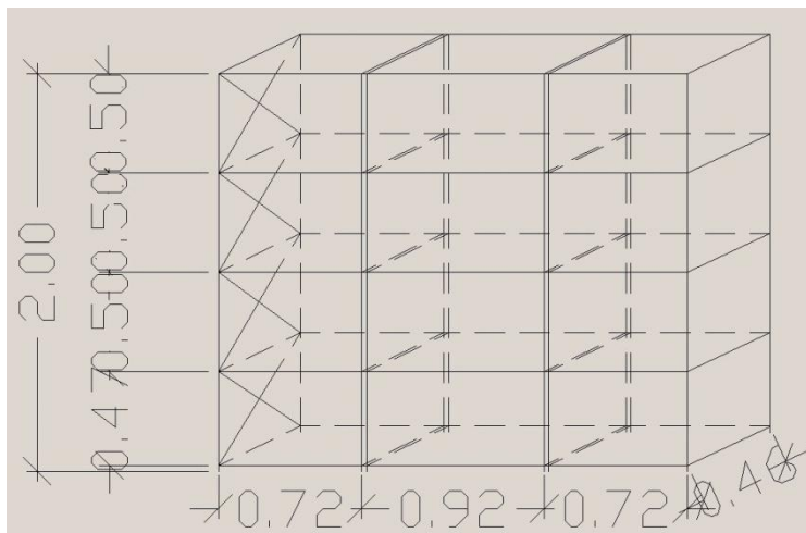
Σχήμα 4. Κατασκευή Γ (dexion)
