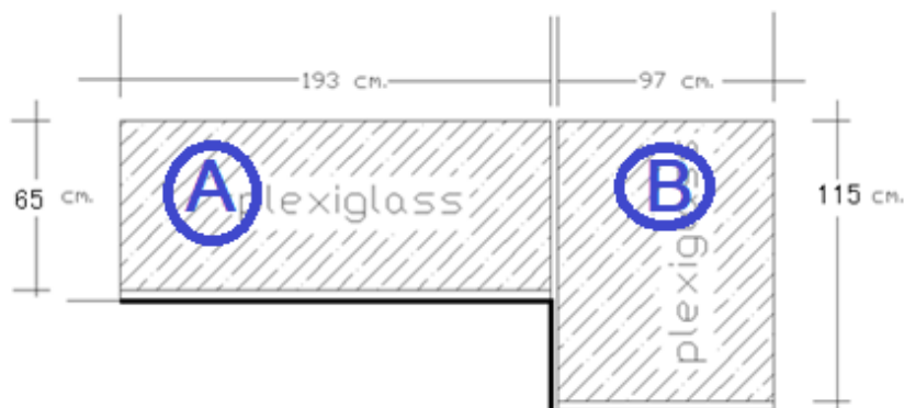
Σχέδιο 1. Προστατευτικό από πλεξιγκλάς για την στάσεις νοσηλευτικής Κεντρικού Κτιρίου
